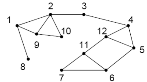
(d) spanning subgraph of G
